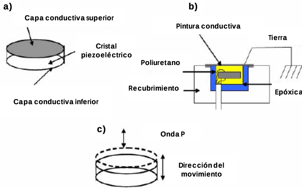
Figura 1.5 Discos Piezoeléctricos: a) Estructura, b) Instalación, c) Funcionamiento, (Valle, 2006)
