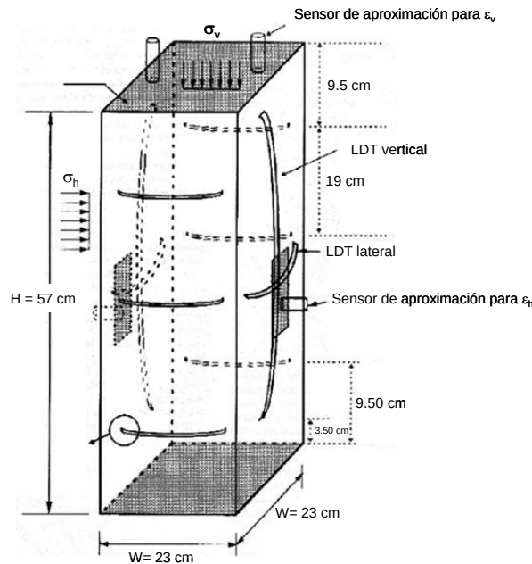
Figura 1.26 Cámara triaxial instrumentada, (Hoque et al. , 1996)
