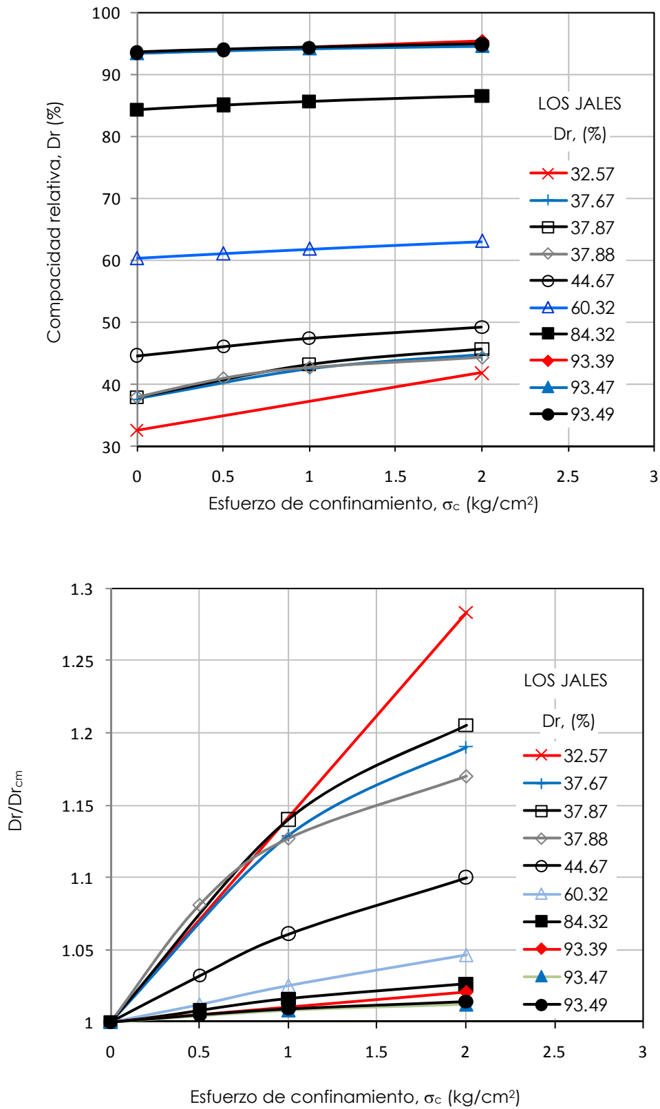
Figura 4.3 Variación de la compacidad relativa inicial con el esfuerzo de confinamiento, Los Jales
