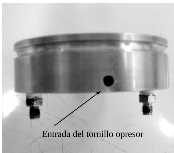
Figura 3.7 Pedestal (perfil)
