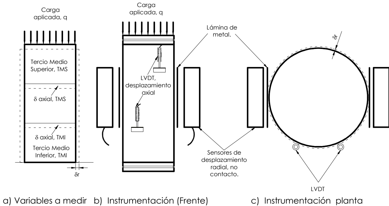
Figura 2.5 Instrumentación de la probeta
