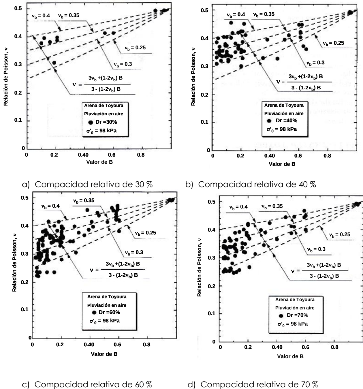
Figura 1.21 Variación de la relación de Poisson con la compacidad relativa y la B de Skempton (Tsukamoto et al., 2002)
