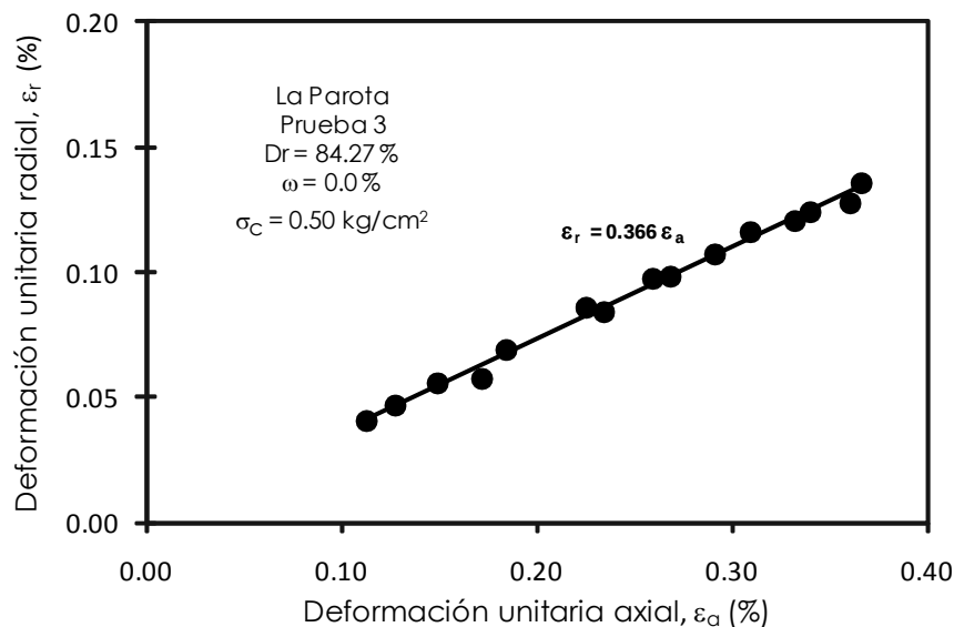
Figura 4.7 Obtención de la relación de Poisson
