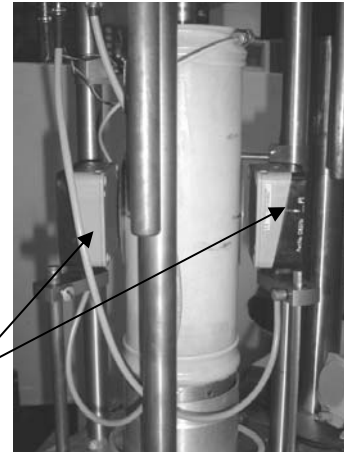
Sensor de desplazamiento radial en el tercio central
