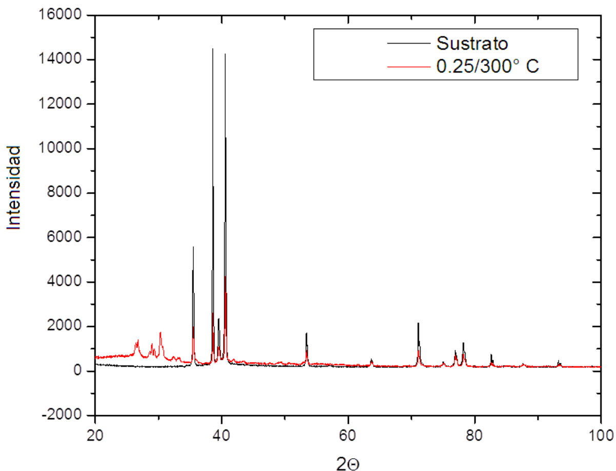
Fig. 4.60 Difractograma del recubrimiento depositado a 300° C con 0.25% vol. de H_3PO_4 y del sustrato.
