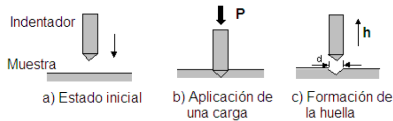
Fig. 2.17 Esquema del proceso de nanoindentación [30].
