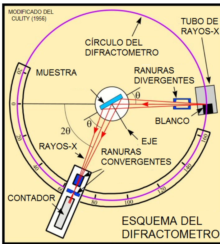
Fig. 2.21 Esquema de un difractómetro de rayos-X [32].
