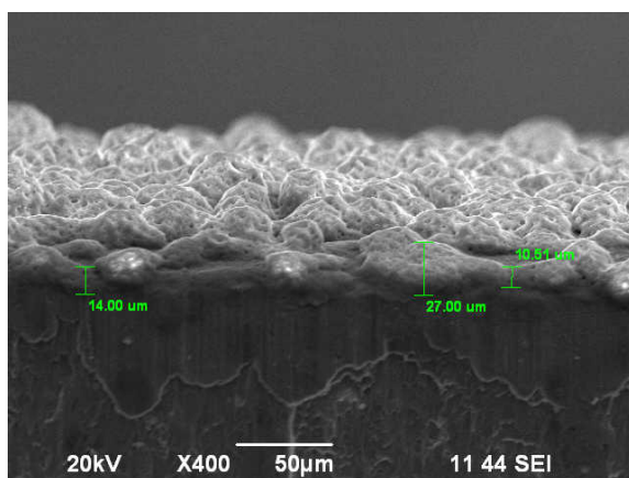
Fig. 4.55 Morfología de la sección transversal del recubrimiento 11a (400X).
