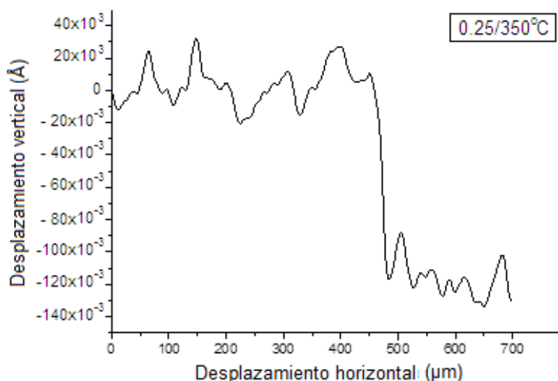
Fig. 4.58 Desplazamiento de la punta del perfilometro correspondiente al perfil lineal de la superficie.
