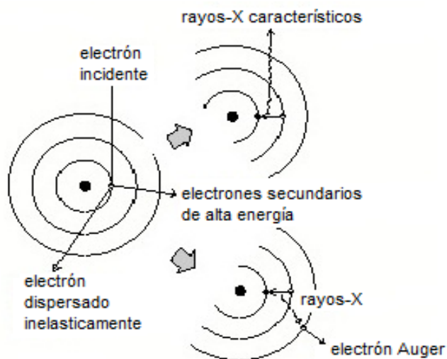
Fig. 2.14 Representación esquemática de la producción de rayos-X y electrones Auger [27].
