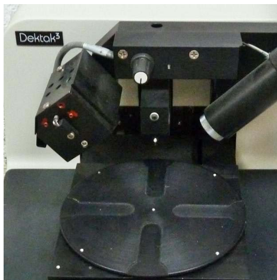
Fig. 3.5 Perfilometro de superficie.
