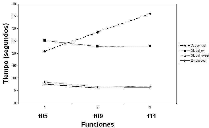
Figura 5.1: Comparativo del desempeño de las variantes PSO en función de la complejidad de la función objetivo
