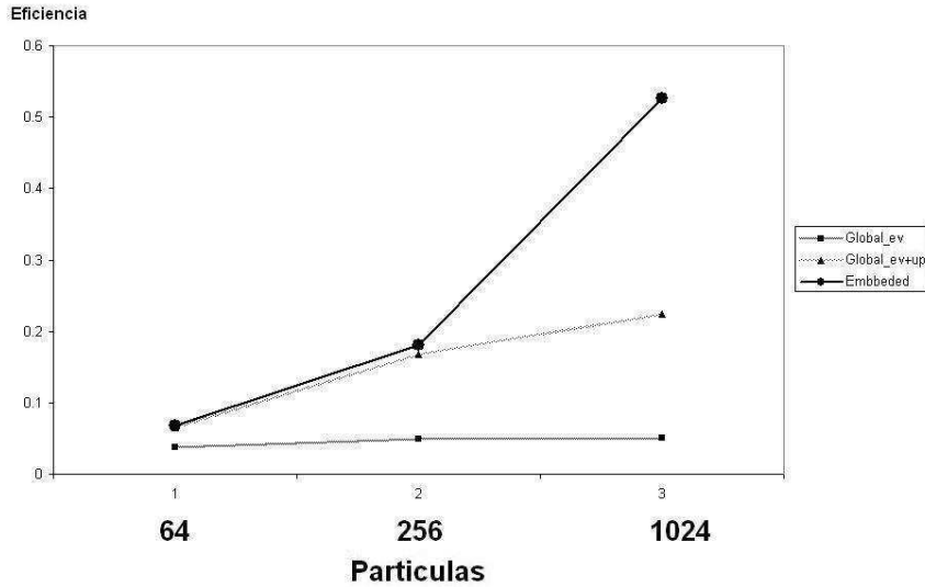
Figura 5.8: Comparativo de la eficiencia de las variantes PSO paralelas en función del número de partículas
