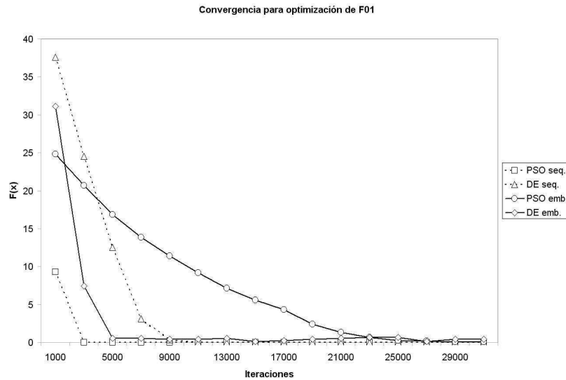
Figura 5.9: Convergencia para optimización en la función F01, con un número fijo de 128 individuos y con iteraciones variables
