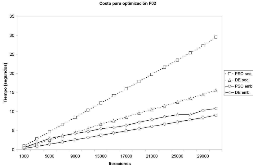
Figura 5.13: Costo en la función F02, con un número fijo de 128 individuos y con iteraciones variables
