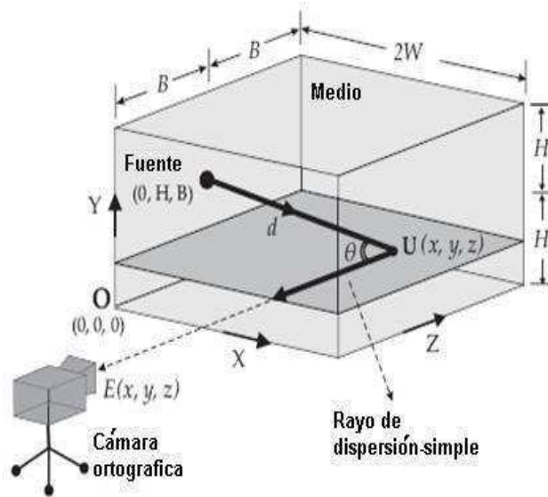
Figura 2.5: Esquema de dispositivo de adquisición de propiedades de dispersión en medios participantes diluidos
