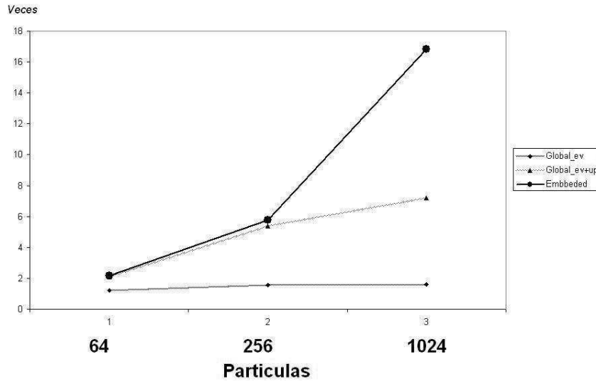
Figura 5.6: Comparativo de la ventaja de las variantes PSO paralelas en función del número de partículas
