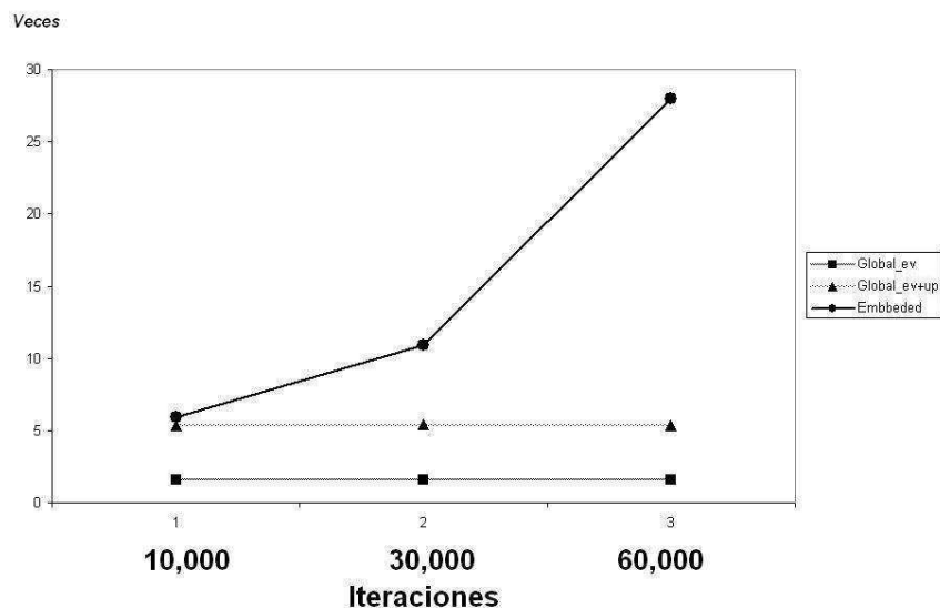
Figura 5.5: Comparativo de la ventaja de las variantes PSO paralelas en función del número de iteraciones
