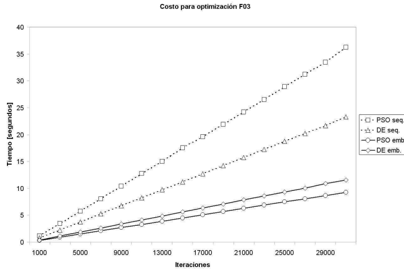
Figura 5.14: Costo en la función F03, con un número fijo de 128 individuos y con iteraciones variables
