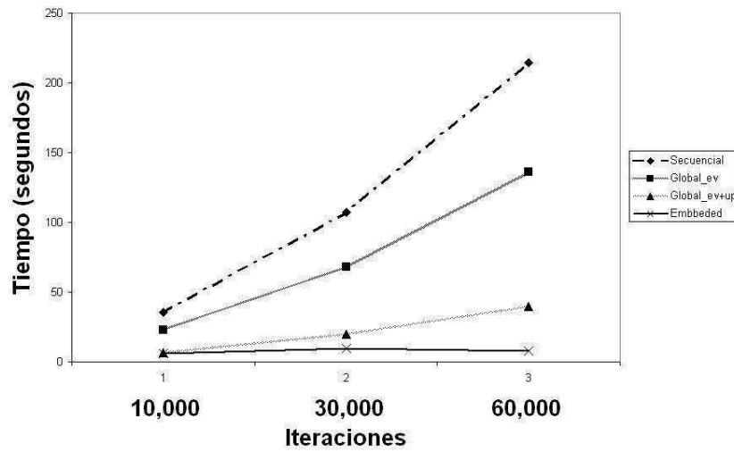
Figura 5.3: Comparativo del tiempo consumido por las variantes PSO, en función del número de iteraciones, para la optimización de F11
