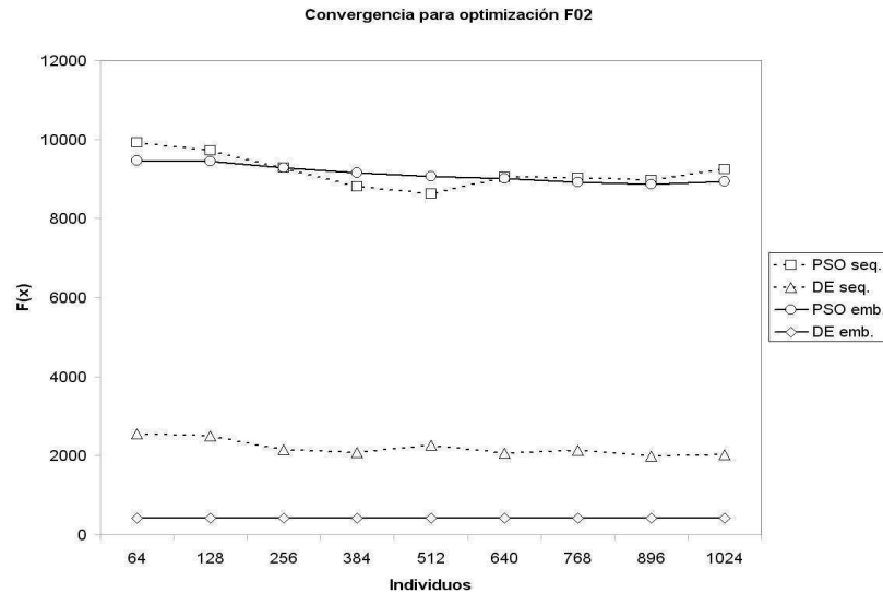
Figura 5.16: Convergencia para optimización en la función F02, con un número fijo de 2000 iteraciones y con número de individuos variable
