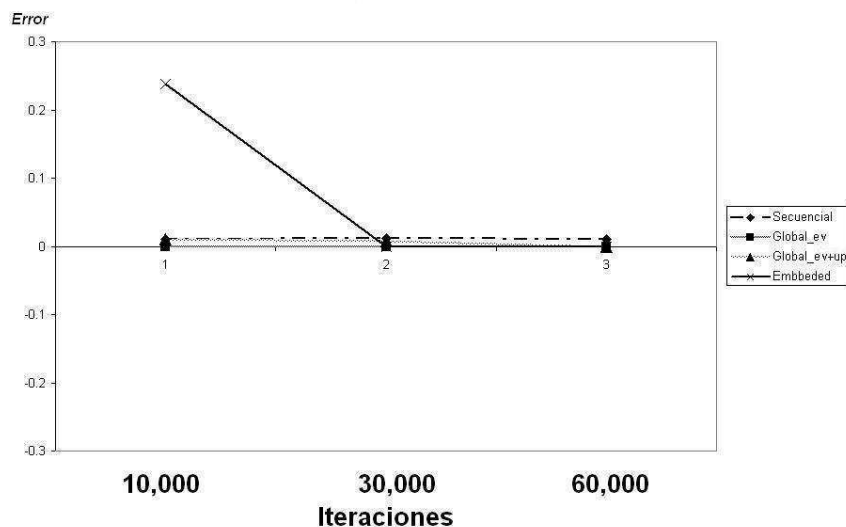
Figura 5.2: Comparativo del error de las variantes PSO, en función del número de iteraciones, para la optimización de F11
