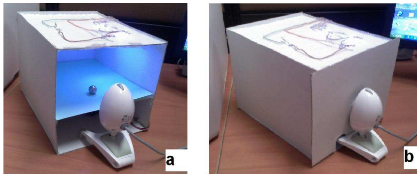
Figura 4.5: Sistema de adquisición de imágenes de referencia
