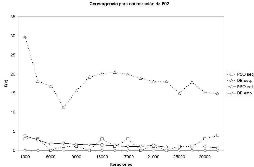
Figura 5.10: Convergencia para optimización en la función F02, con un número fijo de 128 individuos y con iteraciones variables
