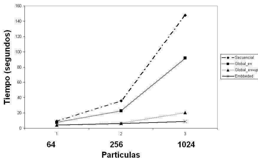
Figura 5.4: Comparativo del tiempo consumido por las variantes PSO, en función del número de partículas, para la optimización de F11
