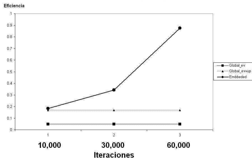
Figura 5.7: Comparativo de la eficiencia de las variantes PSO paralelas en función del número de iteraciones
