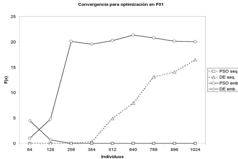
Figura 5.15: Convergencia para optimización en la función F01, con un número fijo de 2000 iteraciones y con número de individuos variable
