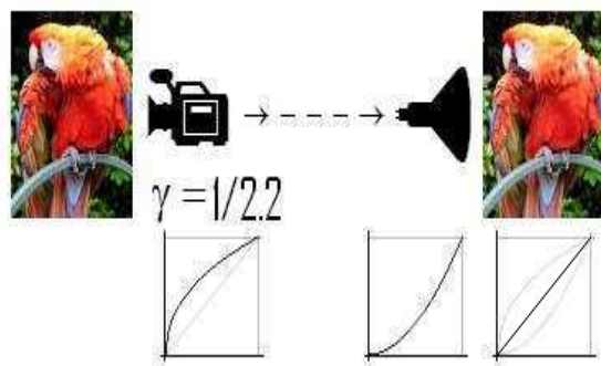
Figura D.2: Imagen lineal mostrada en un dispositivo con comportamiento no lineal y con corrección gamma
