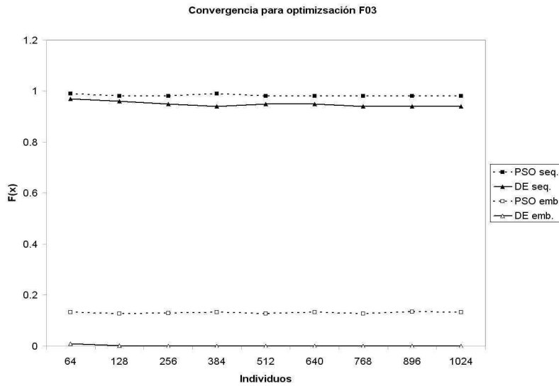
Figura 5.17: Convergencia para optimización en la función F03, con un número fijo de 2000 iteraciones y con número de individuos variable
