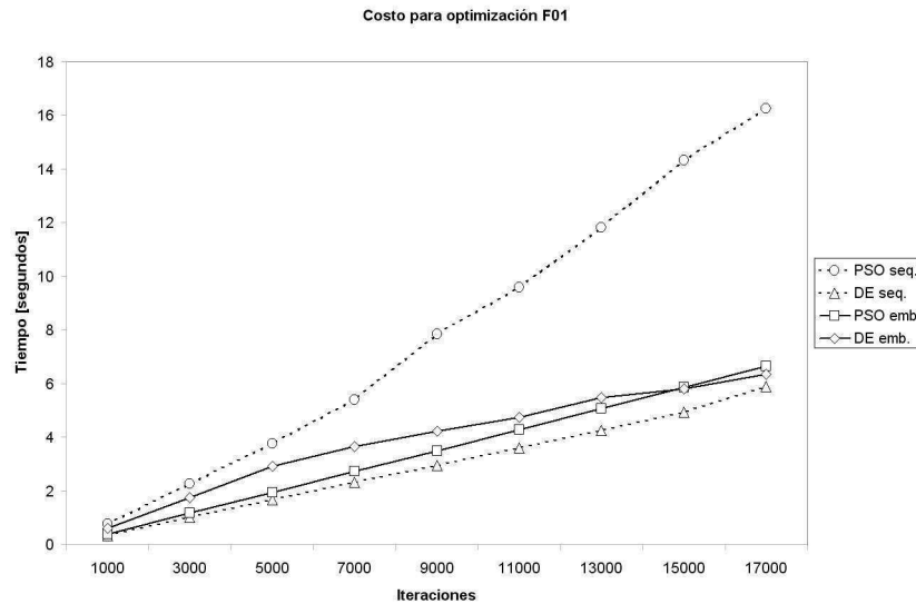
Figura 5.12: Costo en la función F01, con un número fijo de 128 individuos y con iteraciones variables
