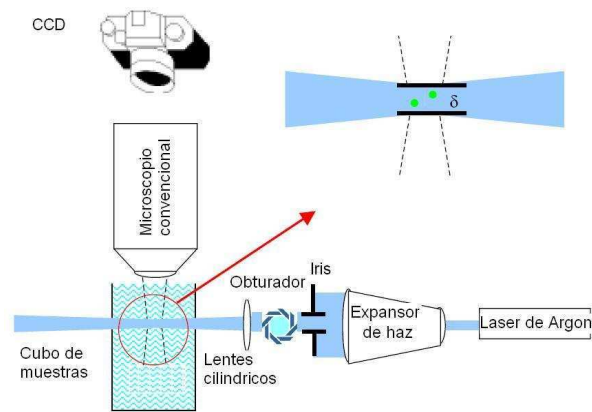
Figura 2.3: Un microscopio de hoja delgada de luz laser para oceanografía microbiana, Fuchs et al.
