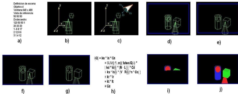
Figura B.2: Etapas del proceso de renderizado: a) Definición de escena, b) Conformación de la escena, c) Definición del punto de vista, d) Antes de eliminar los polígonos ocultos, e) Polígonos ocultos eliminados, f) Recorte a volumen 3D, g) Eliminación de superficies ocultas, h) Modelo de iluminación, i) Rasterización, j) Despliegue de la imagen.
