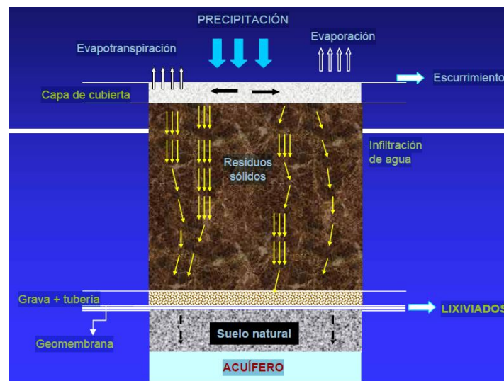
Figura 11. Generación de lixiviados en relleno sanitario 30
