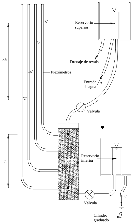
Figura 23. Permeámetro de carga constante.
