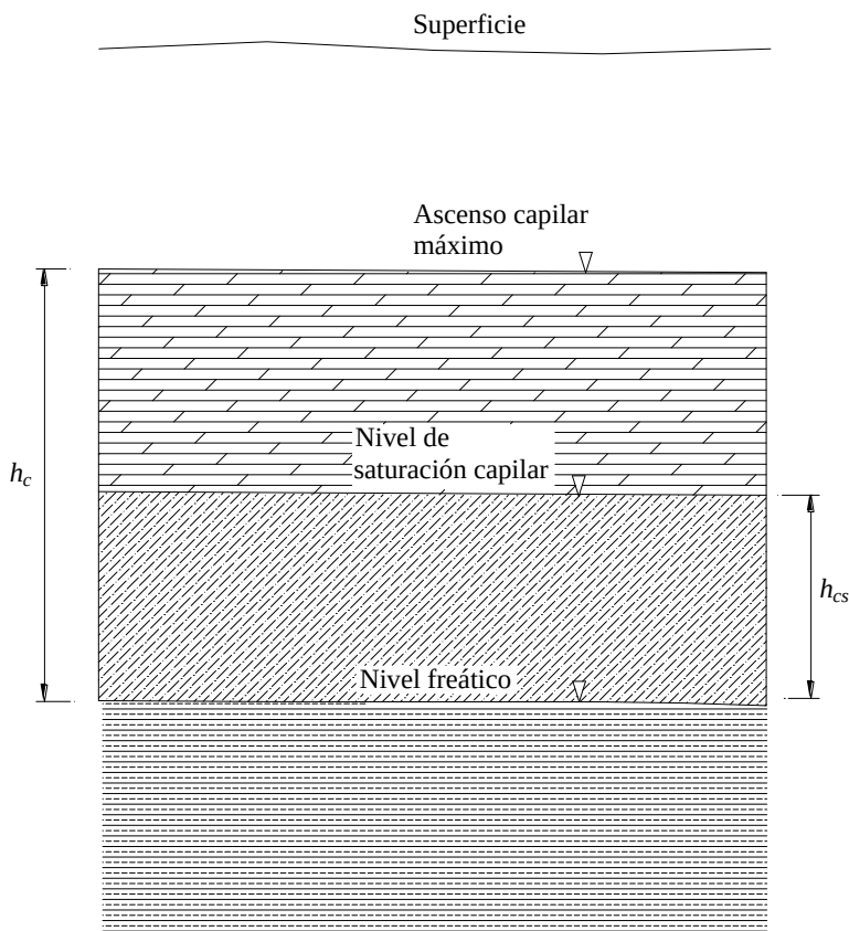
Figura 22. Ascensión capilar de agua en el suelo.
