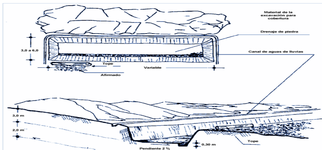
Figura 6. Método de trinchera para construir un relleno sanitario 10
