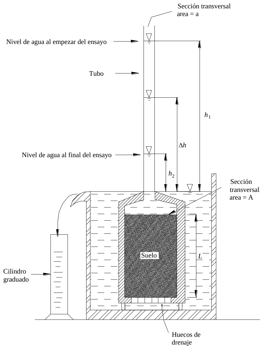
Figura 24. Permeámetro de carga variable.
