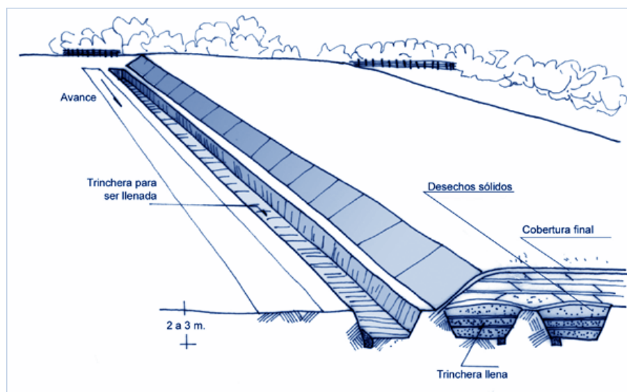
Figura9. Combinación de ambos métodos para construir un relleno sanitario 12
