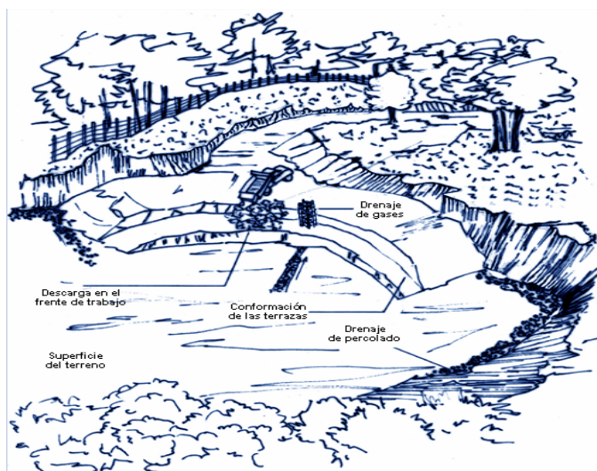
Figura 8. Método de área para rellenar depresiones 10
