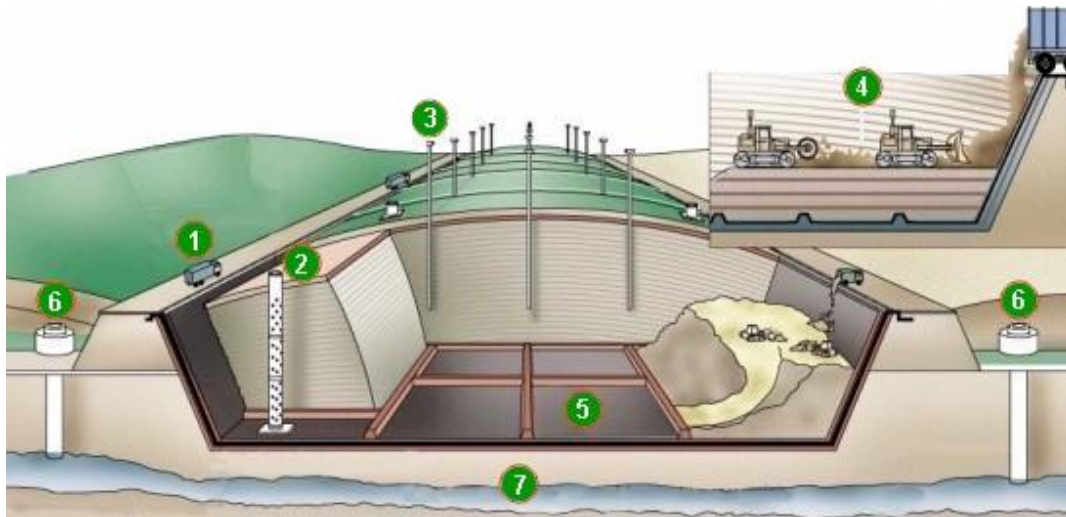
Figura 10. Funcionamiento de un relleno sanitario
