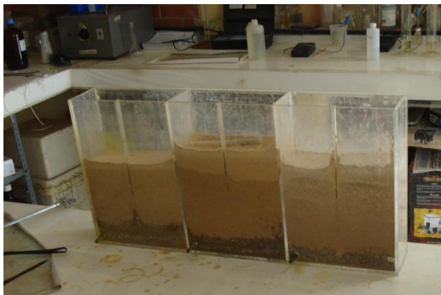
Figura 33. Acrílico con suelo compactado en 3 secciones para la prueba de permeabilidad
