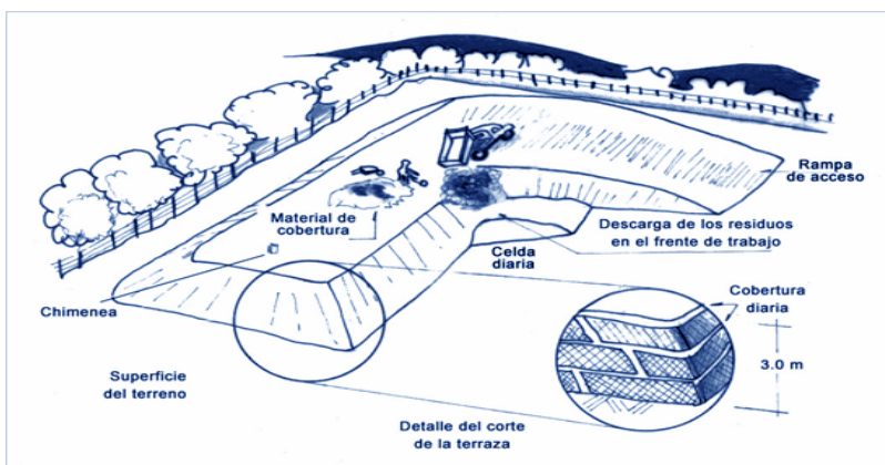
Figura 7. Método de área para construir un relleno sanitario 11
