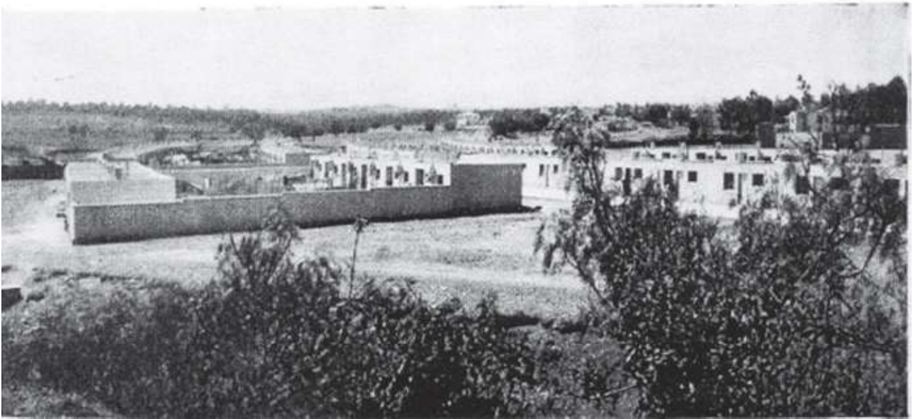
Casas unifamiliares de propiedad privada, Col. Obrera de Balbuena y Col. Obrera de las Lomas de Chapultepec, México, DF. Fuente: revista Arquitectura , selección de arquitectura, urbanismo y decoración. No. 12. Abril de 1943.
