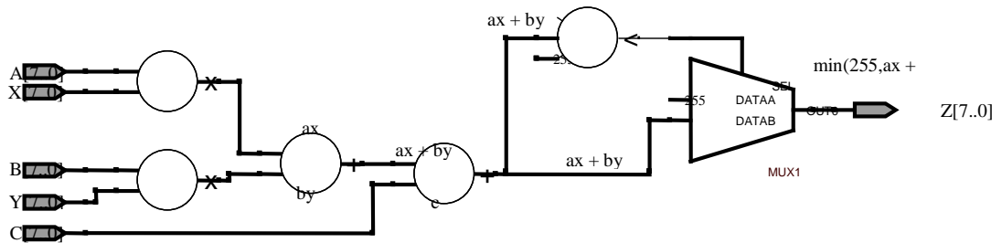
Figura 3.10. Diagrama a bloques de la función de salida para sistema Sugeno. a) Diagrama lógico del valor de certero del conjunto de salida sugeno, b) diagrama de boque de las 9 funciones de salida.
