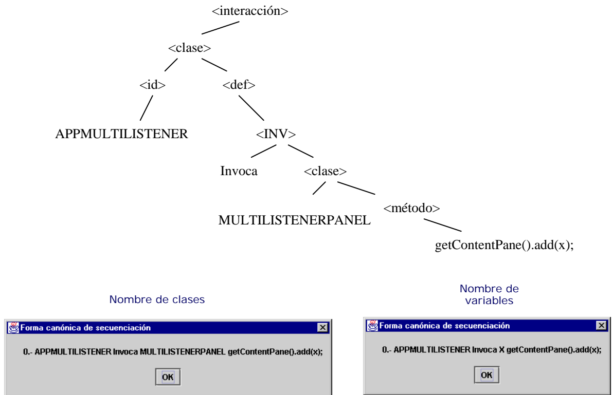
Figura 5.6 Árbol de derivación
