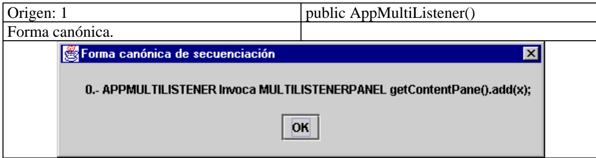
Figura 5.5 Forma canónica para el origen número 1.
