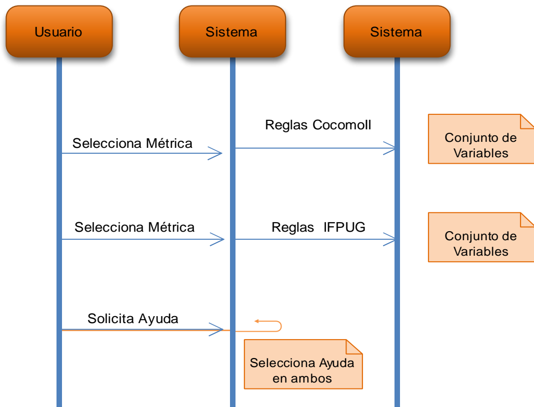
Figura 2. Diagrama de Secuencia de las fases de la Aplicación.
