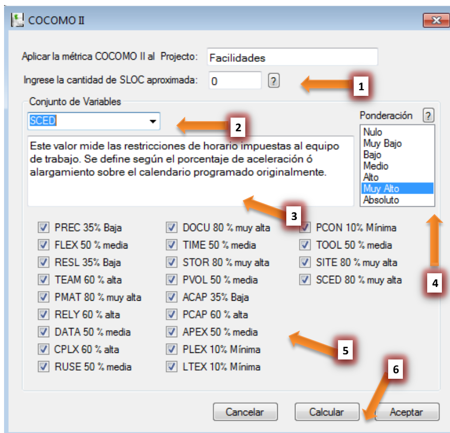
Figura 10.- Vista del módulo "Evaluación COCOMO".
