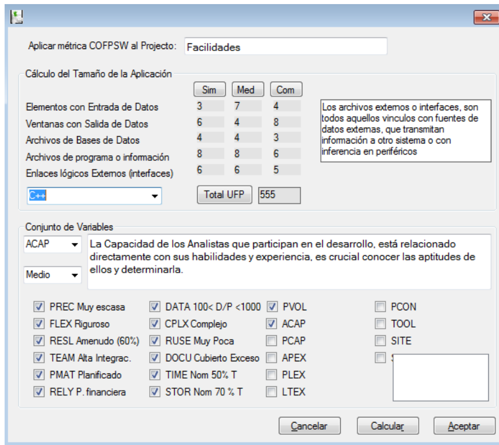
Figura 15.- Vista del módulo de la "Evaluación COFPSW".
