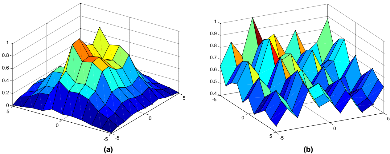
Fig. 4.10 Gráficos en 3D de la distribución de los datos, a) señales blanqueadas y b) señales separadas por ICA
