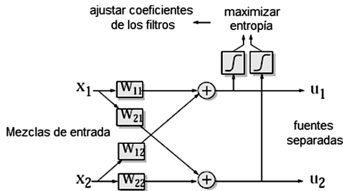
Fig. 4.12 Diagrama de bloques del modelo convolutivo
