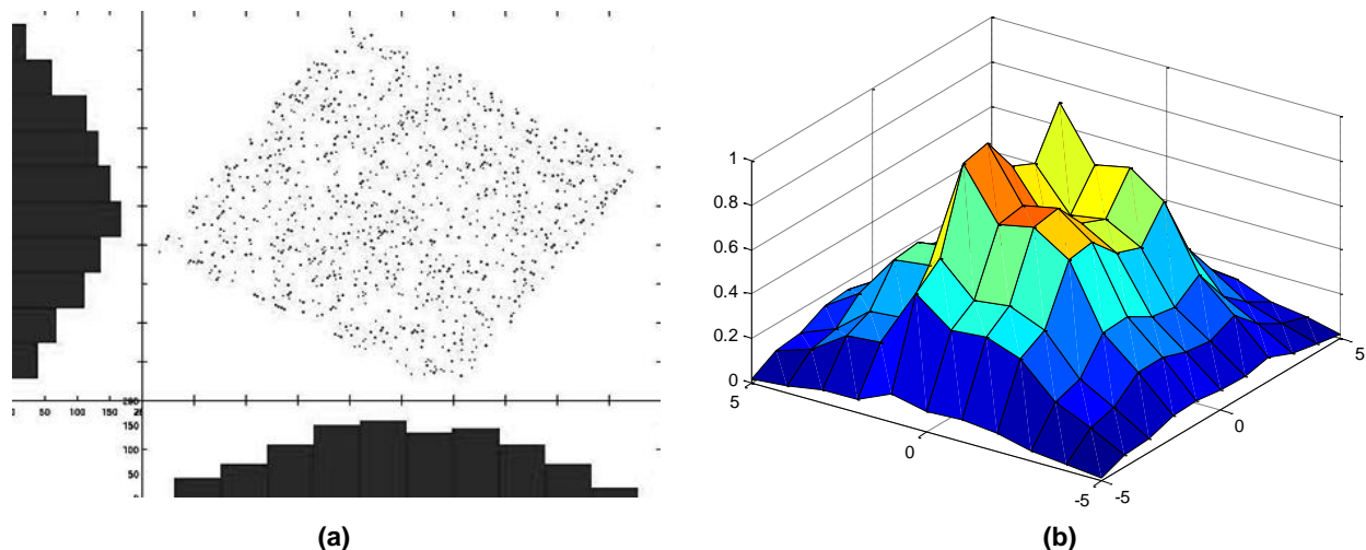
Fig. 3.4 Distribución gaussiana de las señales blanqueadas. a) Histograma de señales mezcladas, b) Gráfico en 3D de la distribución de la mezcla.
