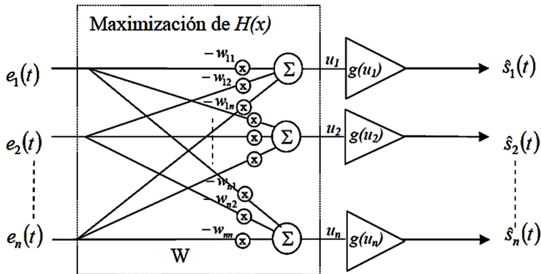
Fig. 3.6 Arquitectura de red neuronal para algoritmo INFOMAX
