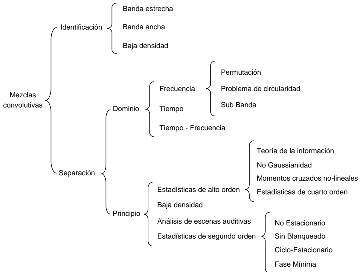
Fig. 2.3 Taxonomía de los métodos más relevantes para separación ciega de mezclas convolutivas.
