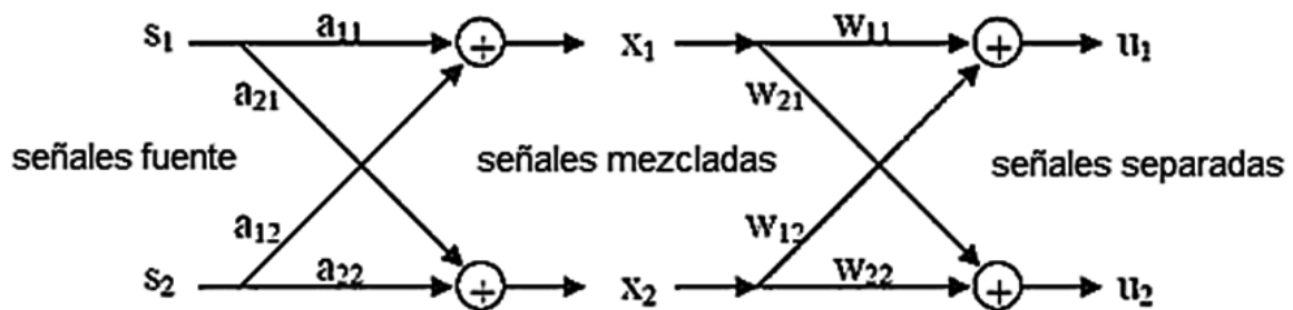
Fig. 4.11 Diagrama de bloques del modelo lineal
