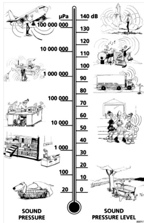
Fig. 2.1 Escala en \mu\text{Pa} comparada con la escala en dB.
