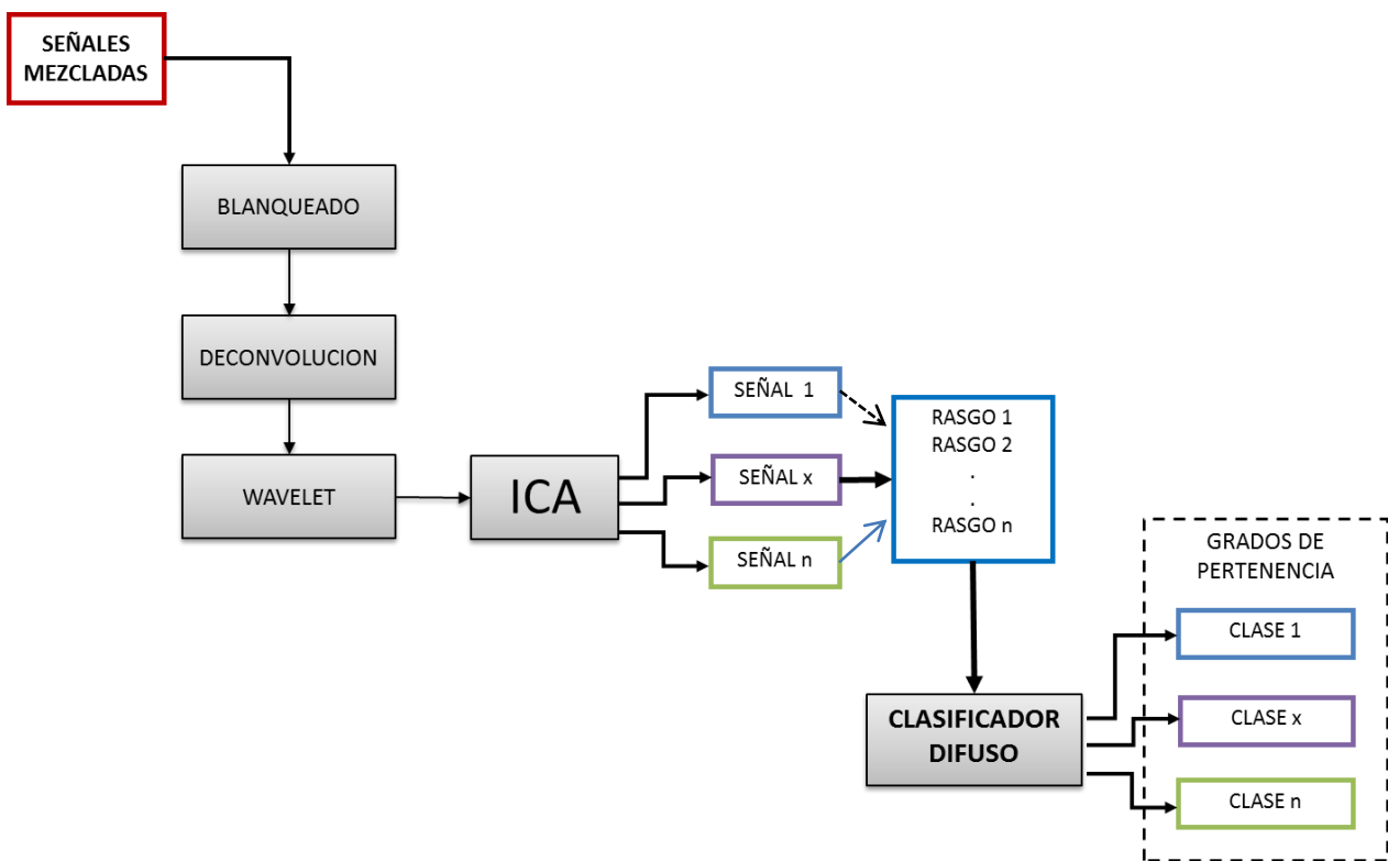
Fig. 4.14 Sistema de separación y clasificación para mezclas reales
