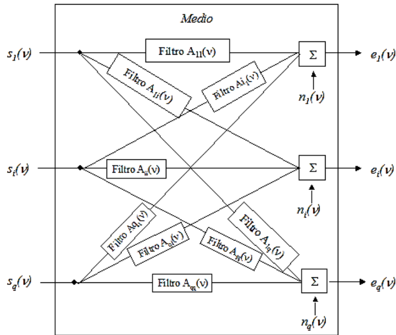
Fig. 3.8 Modelo de mezcla convolutiva
