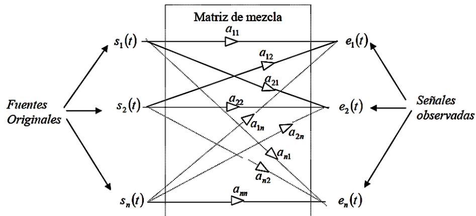
Fig. 3.5 Modelo de mezcla lineal
