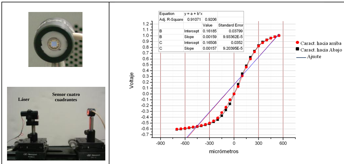
Fig. 8 Sensor óptico PSD
