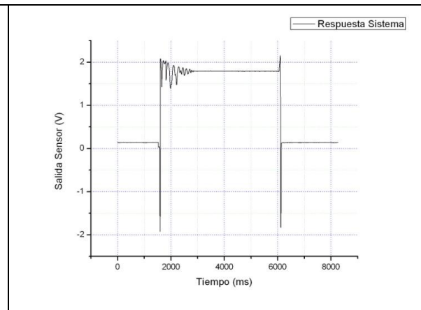
Fig. 14 Respuesta del sistema sintonizado
