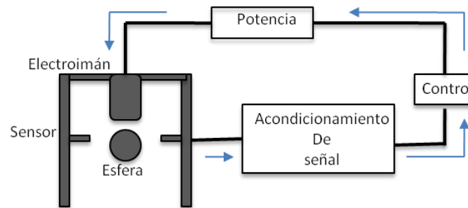
Fig. 1 Sistema de suspensión magnética básico
