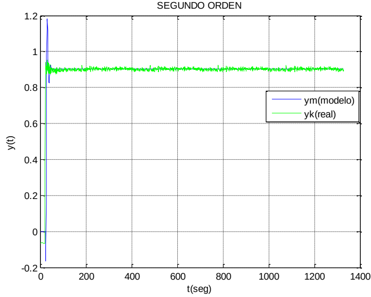
Fig. 5.8 Ajuste de curva con mínimos cuadrados orden 2
