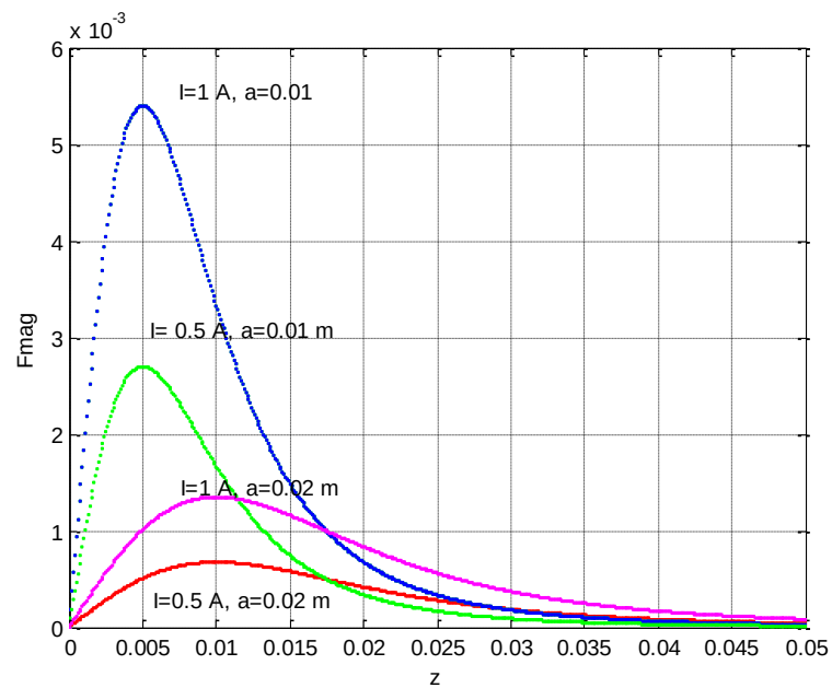
Fig. 4.10 Fuerza magnética con respecto a una distancia
