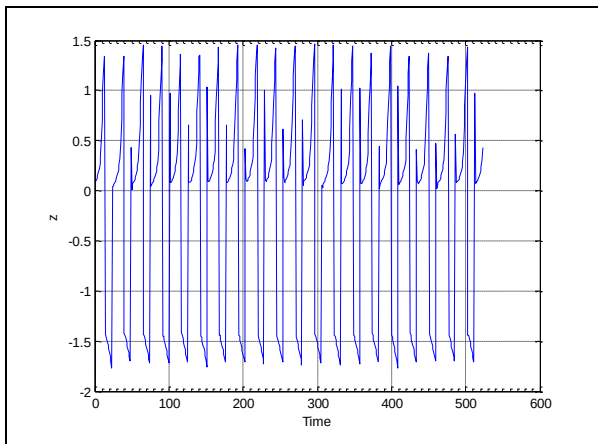
Fig. 13 Respuesta física del sistema K_r=6
