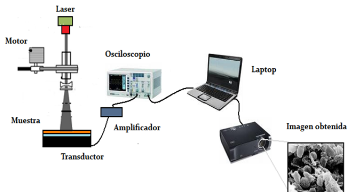
Figura 1. Diagrama del sistema fotoacústico
