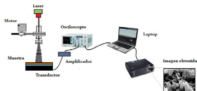
Figura 1. Diagrama del sistema fotoacústico
