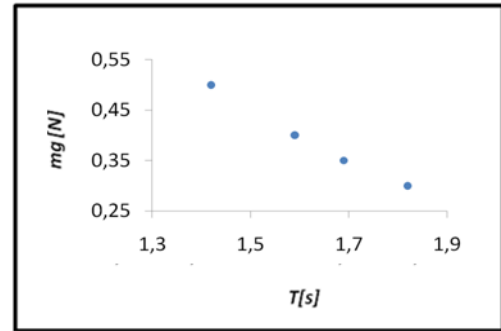
FIGURA 12. Curva de mg vs. T .
