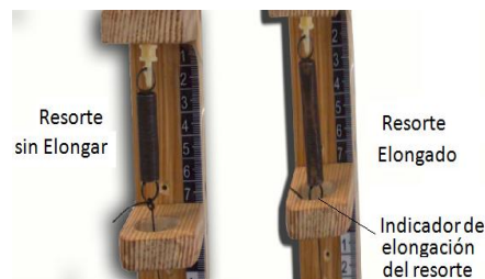
FIGURA 6. Resorte sin elongar y elongado por efecto de la masa ( m ) o un movimiento circular uniforme.
