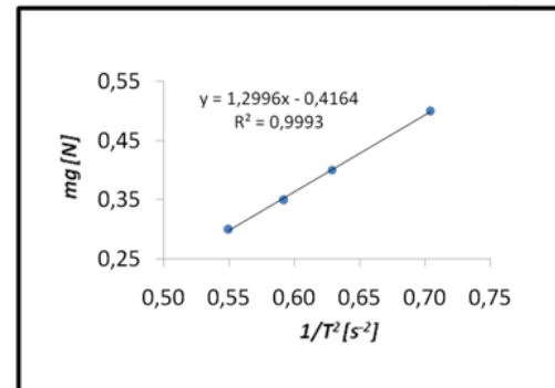
FIGURA 13. Curva de mg vs. \frac{1}{T^2}
