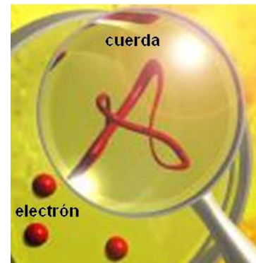
FIGURA 3. Diversos modos de vibración representan una partícula diferente. El tamaño de las cuerdas es muy pequeño ( 10^{-33} cm), mucho más pequeño que el electrón.
